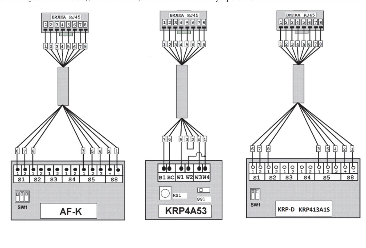
Рисунок 2 Схема соединения СРК-D, СРК-DM с внешними устройствами
