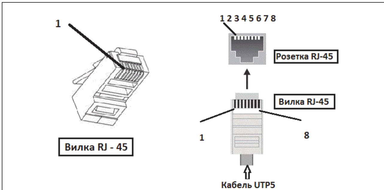
Рисунок 5 Стандартная схема разъёмного соединения RJ-45
