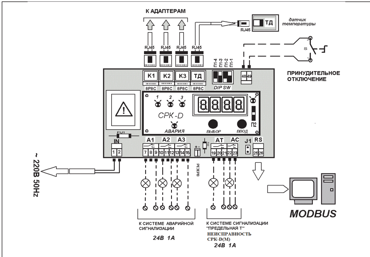
Рисунок 4 Схема для подключения соединительных кабелей к CPK3-D(DM)
